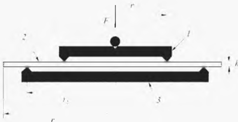
1 – нагружающее кольцо; 2 – образец; 3 – опорное кольцо
