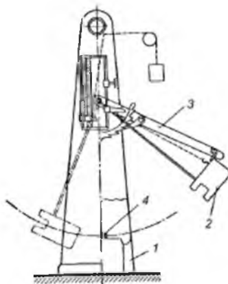
1 – стойки; 2 – маятник; 3 – подъемная рама; 4 – образец
