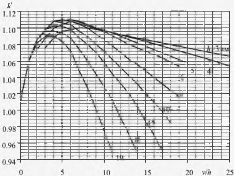
Рисунок 3 – Безразмерный коэффициент k_0 как функция от y/h
