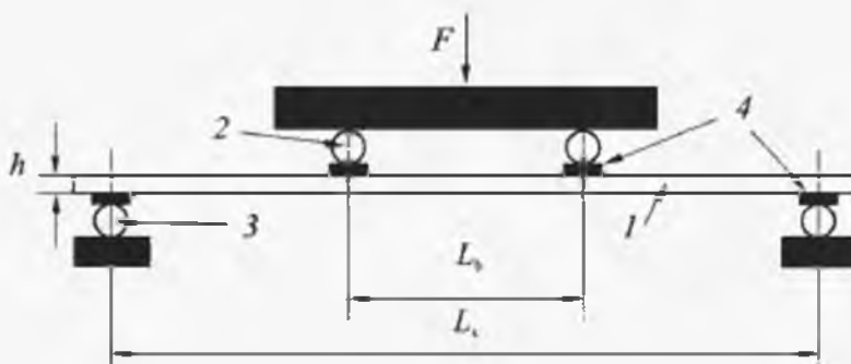
1 - образец; 2 - изгибающие ролик; 3 - опорный ролик; 4 - резиновые полоски. L_b = 200 мм ± 1 мм, L_s = 1000 мм ± 2 мм
